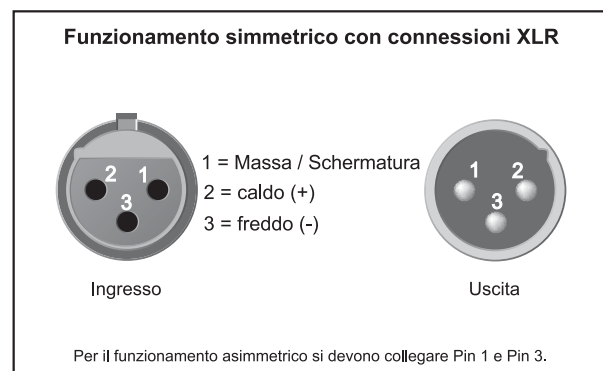
Fig. 4.1: Connettori XLR
